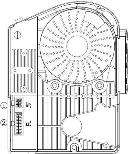
Рис 1. A2 – разъёмы блока управления
